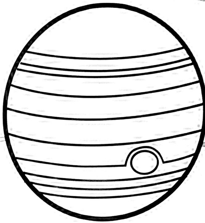
Jupiter
