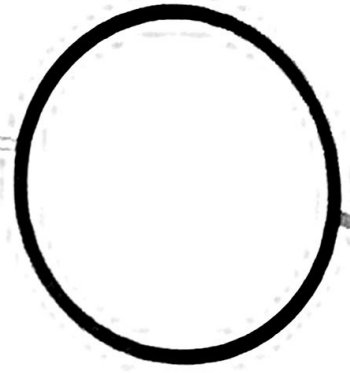
Uranus
