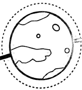
Mars
